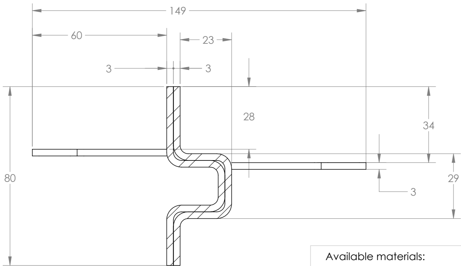
SECTION J SCALE 1 : 1
