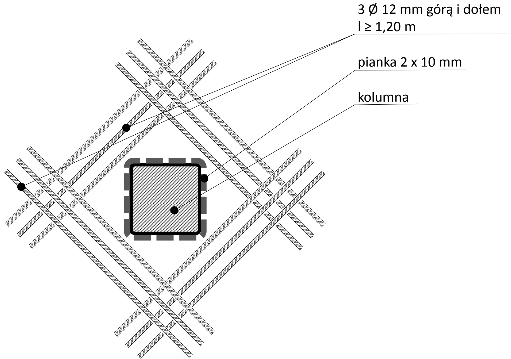
Kolumna centralnie bez dylatacji
