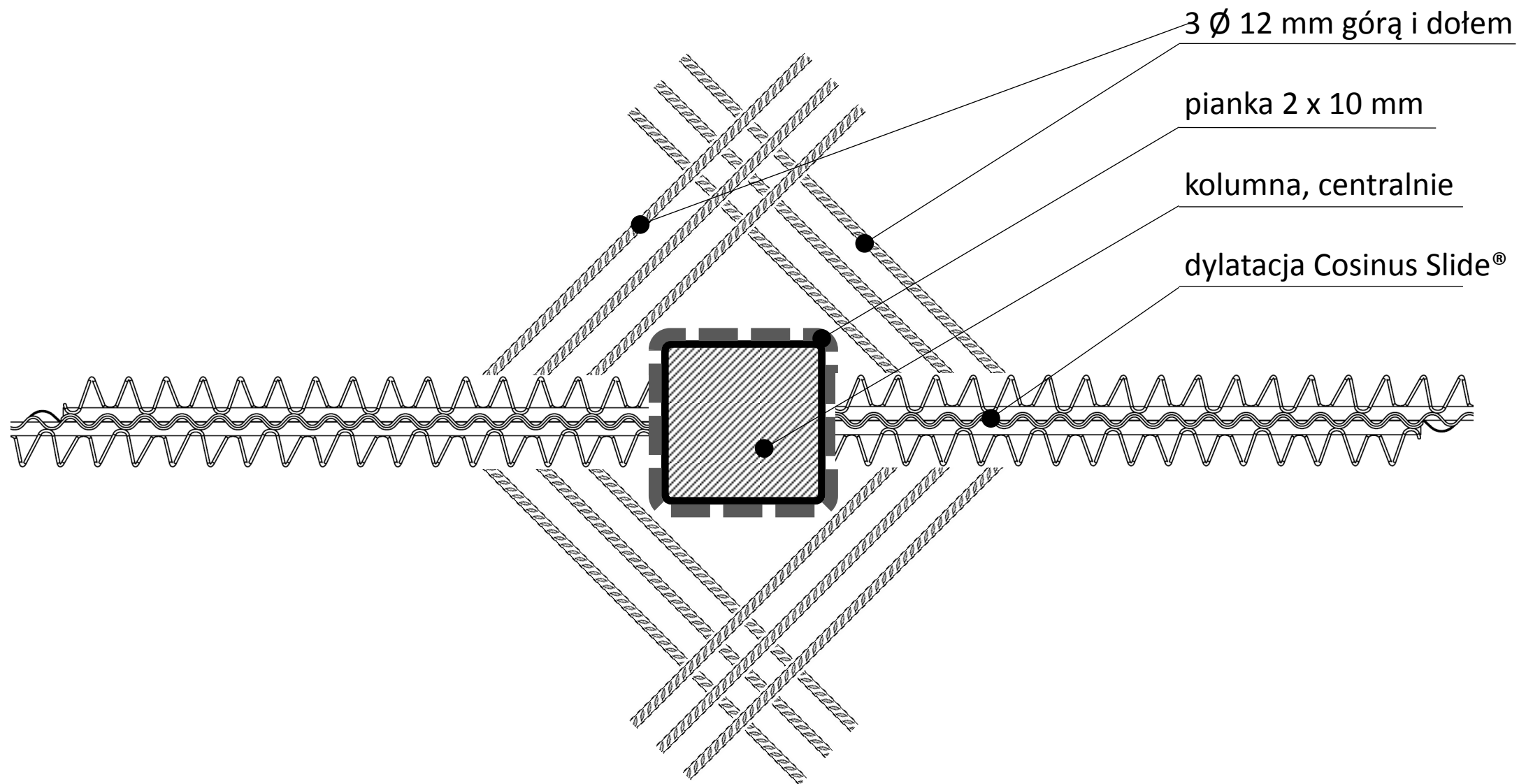
Kolumna centralnie z dylatacjami
